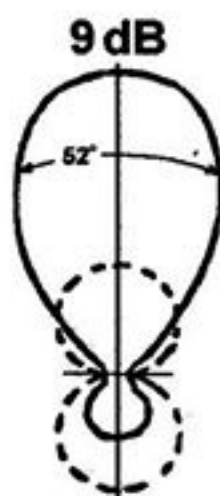
DIAGRAMA DE IRRADIAÇÃO HORIZONTAL
