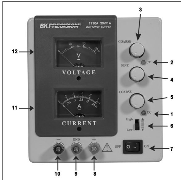
Figura 1. Controles y indicadores de el panel delantero
