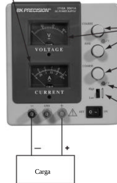
Figura 6. Tipica operación de corriente
