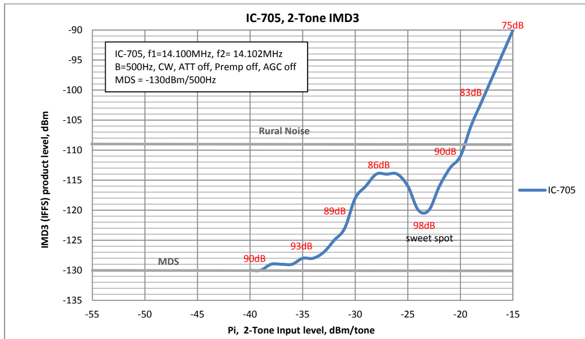
Bild 5: IMD3-Verlauf des IC-705, max. Dynamik im Sweet-Spot: 98dB
