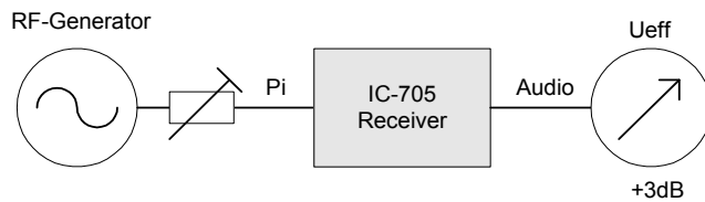
Bild 1: Messaufbau zur Ermittlung der Empfindlichkeit
