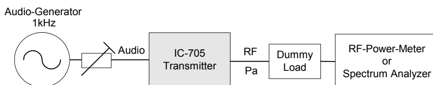
Bild 8: Leistungsmessung mit einem CW-Signal
