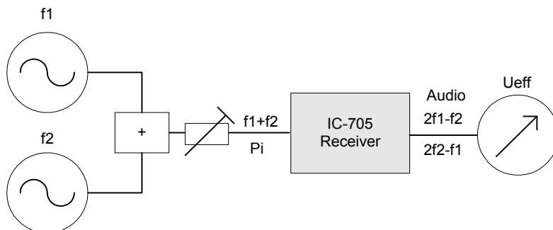
Bild 4: Testaufbau für IMD3-Messung
