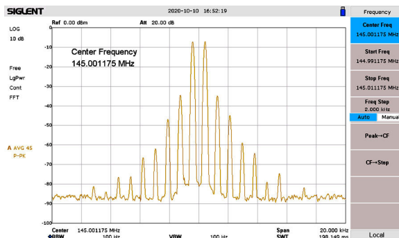
Bild 13: 145MHz, IMD3=30dB
