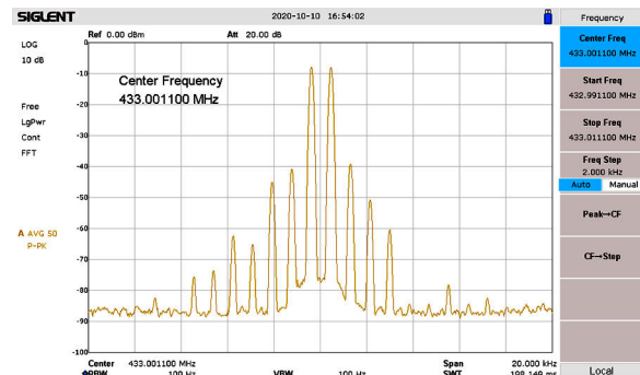
Bild 14: 433MHz, IMD3=32dB
