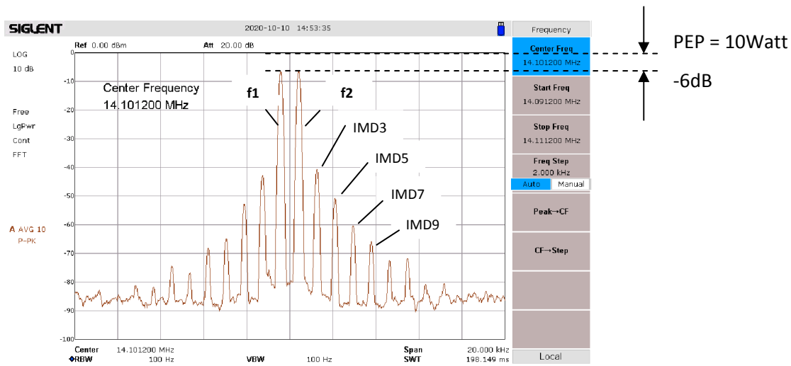
Bild 12: 14.1MHz: IMD3=35dB
