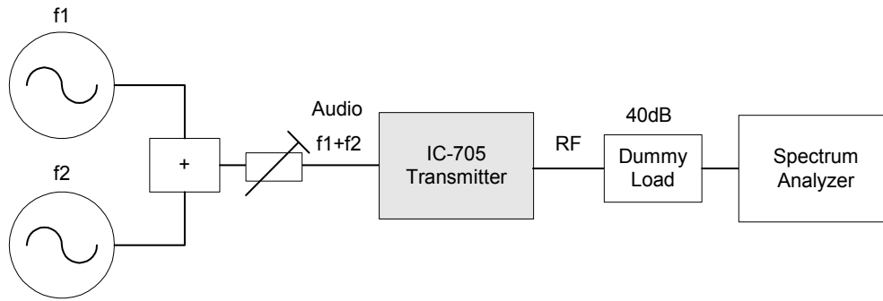
Bild 11: Transmitter IMD-Messung
