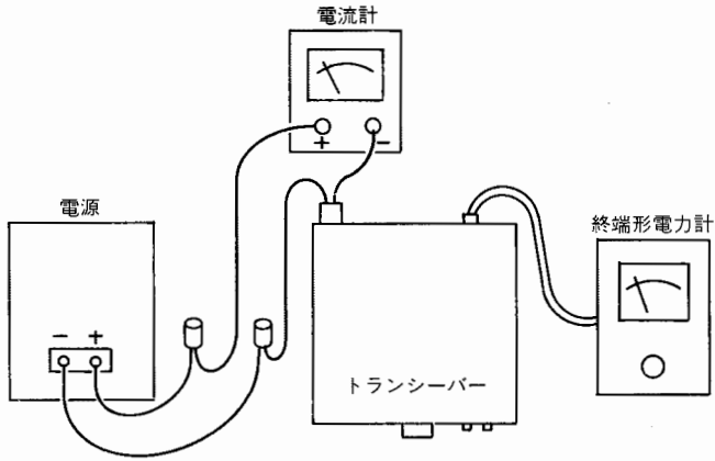
[接続例]
