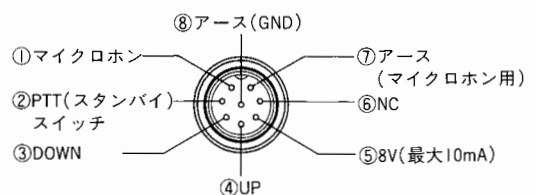
(参考)マイクロホン端子の接続図(前面パネルから見た図)
