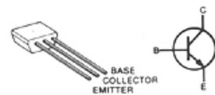
2SC2458-Y Q2001
