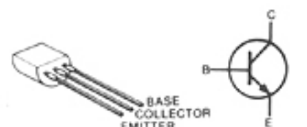
2SC1571G Q1010
