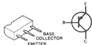
2SB909M Q Q2002
