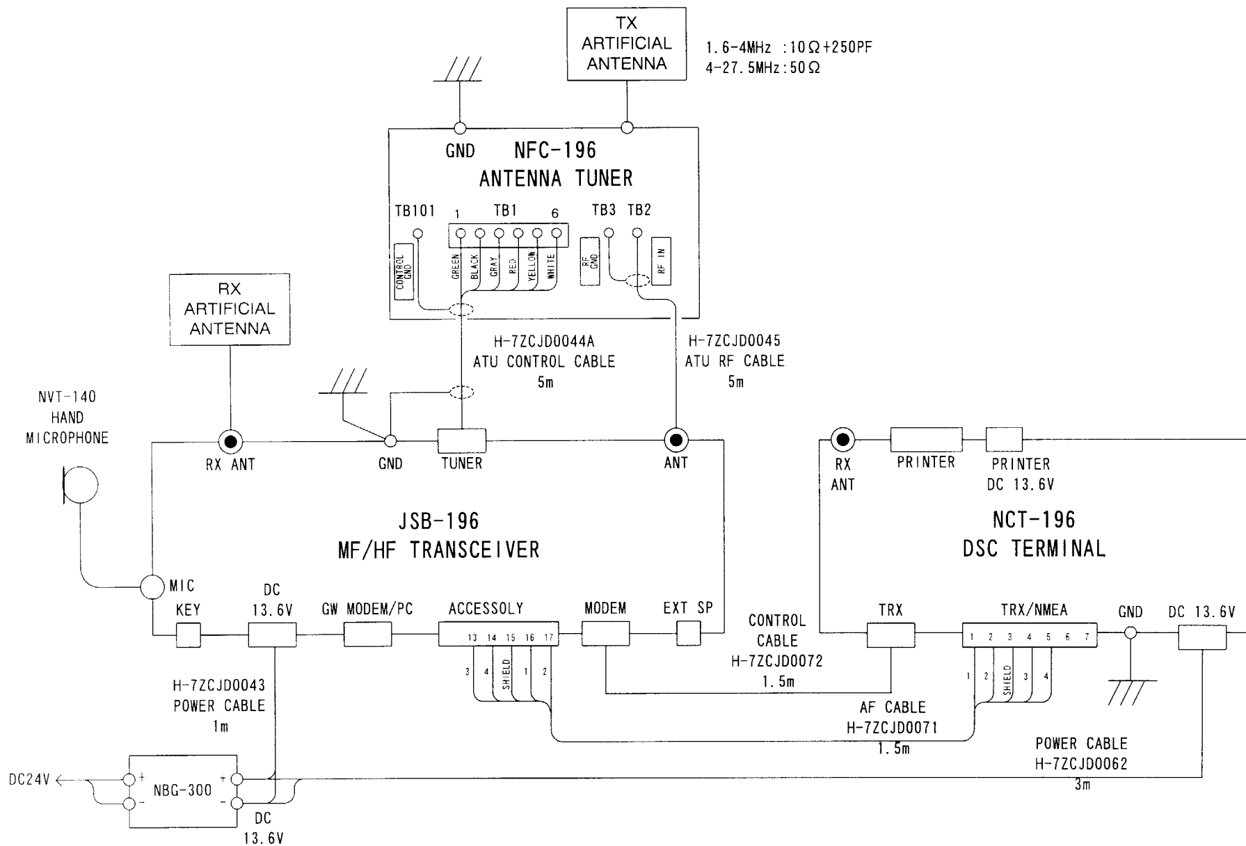
JSB-196GM TEST CONFIGURATION
