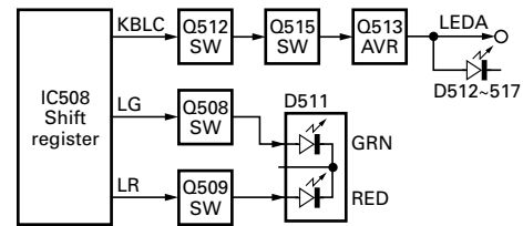
Fig. 10 Display circuit
