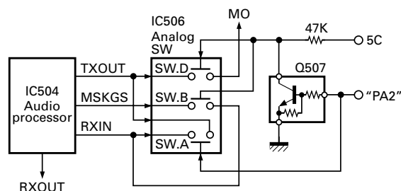
Fig. 15 PA switch
