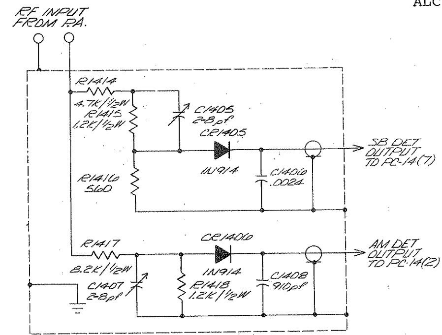
ALC DETECTOR
