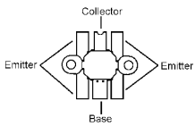
2SC5125 (Q1507)
