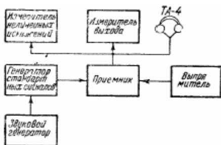
Рис. 28. Блок-схема измерения коэффициента нелинейных искажений.
