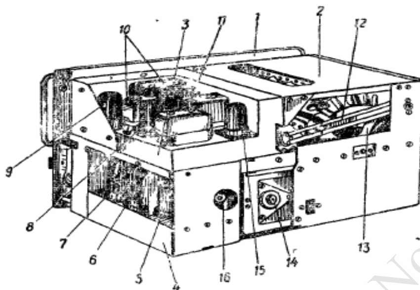
Рис. 15 Вид радиоприемника без кожуха. 1—передняя панель; 2—блок В. Ч; 3—блок П. Ч; 4—блок Н. Ч; 5—лампа Л 11 ; 6—лампа Л 12 ; 7—лампа Л 13 ; 8—лампа Л 14 ; 9—лампа Л 15 ; 10—фильтр промежуточной частоты; 11—лампа Л 16 ; 12—тяга под- стройки антенны; 13—барабанный переключатель; 14—блок конден- саторов переменной емкости; 15—лампа Л 17 ; 16—контур 2-го гетеро- дина
