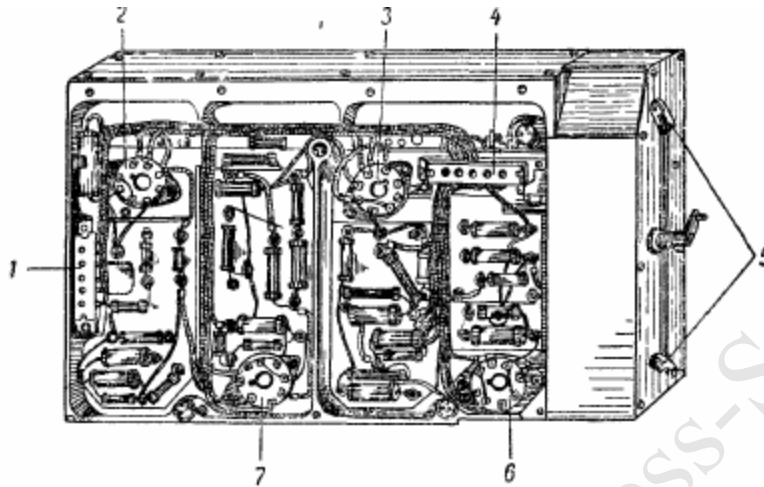
Рис. 21 Блок «ПЧ»; 1—штепсельный разъем; 2—лампа Л 10 ; 3—лампа Л 8 ; 4—штепсельный разъем; 5—конденсаторы С 175 и С 184 ; 6—лампа Л 1 ; 7—лампа Л 9 .
