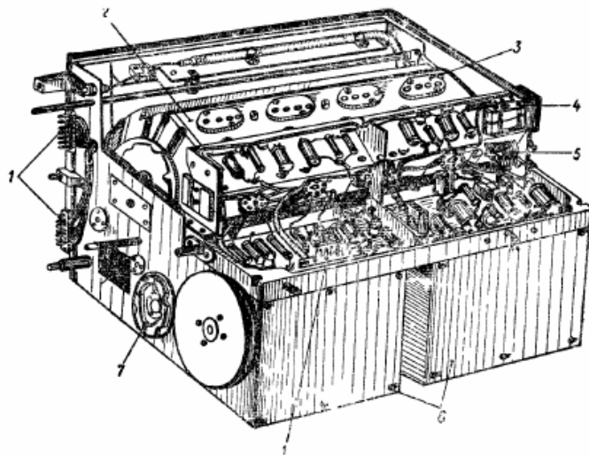
Рис 19. Блок «В4» 1—штепсельный разъем, 2—барабанный переключатель, 3—контактная группа; 4—режекторный фильтр, 5—конденсатор подстройки антенны, 6—блок переменной емкости; 7—ведущая шестерня
