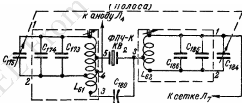
Рис. 8. Кварцевый фильтр.
