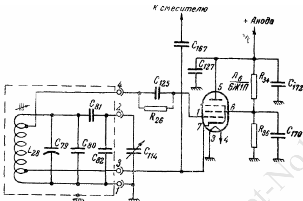
Рис 6 Первый гетеродин
