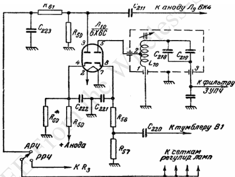
Рис. 9. Детектор сигнала и детектор АРЧ.
