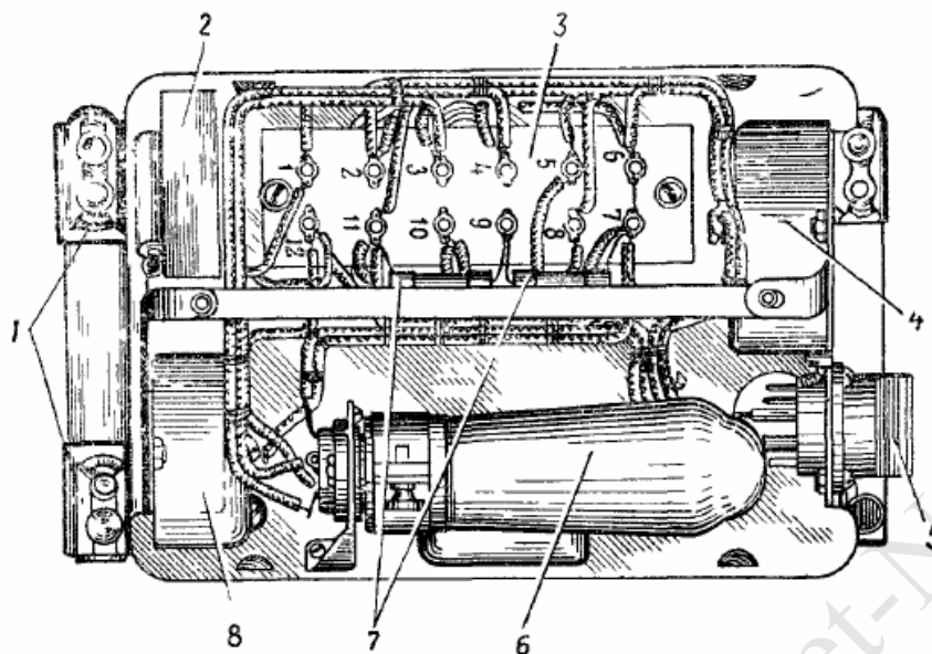
Рис. 23 Блок «В»
