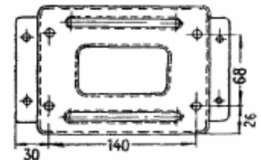
РАМА ВЫПРЯМИТЕЛЯ
