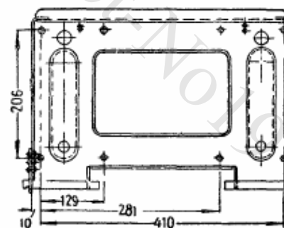
РАМА ПРИЕМНИКА
