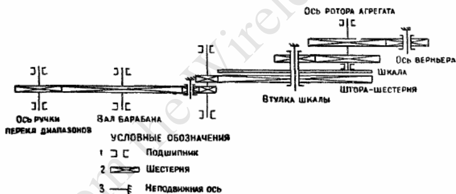
Рис. 24 Кинематическая схема элементов переключения и настройки
