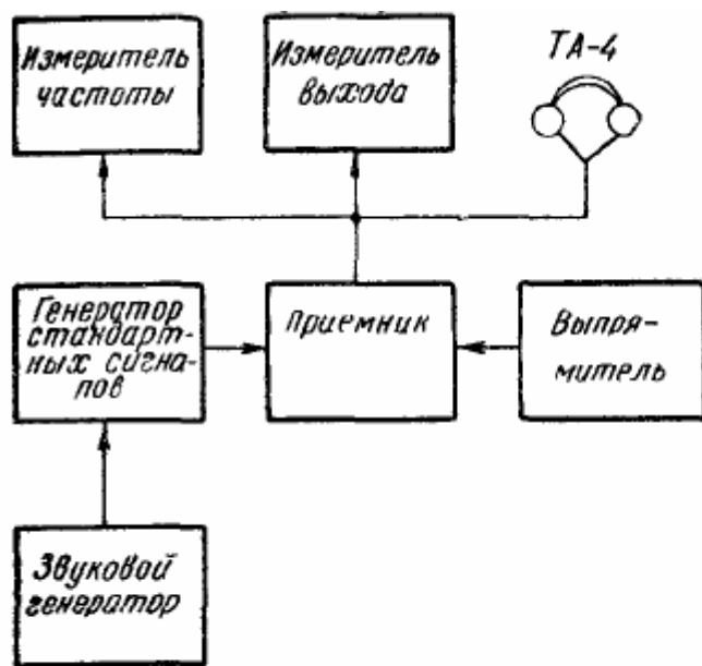
Рис. 25. Блок-схема измерения чувствительности приемника.
