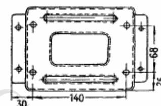
РАМА ВЫПРЯМИТЕЛЯ
