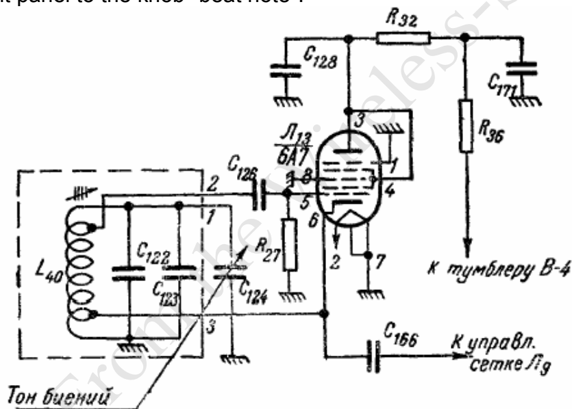
Рис. 11. Второй гетеродин
