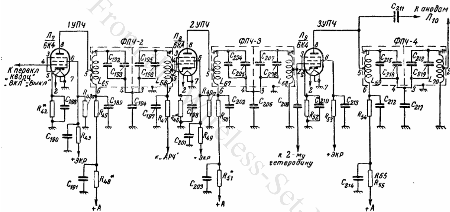
Рис. 7. Усилитель промежуточной частоты.
