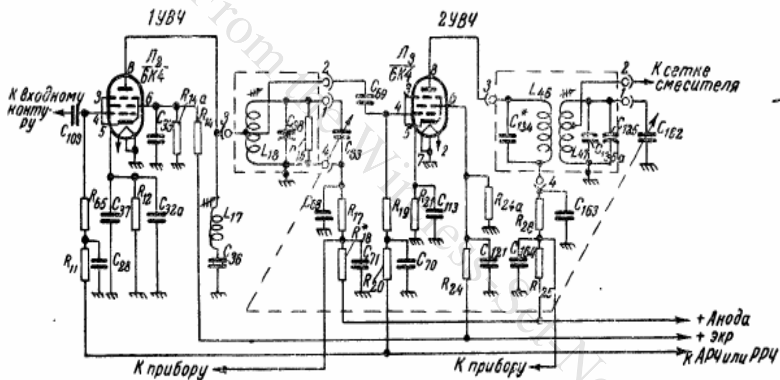
Рис. 30. Усилитель высокой частоты до изменения.
