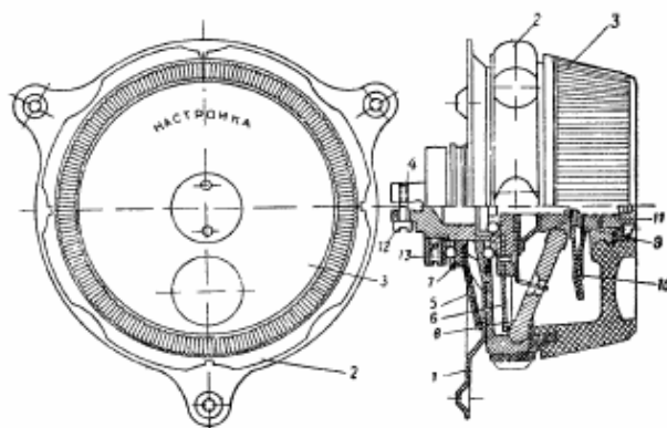
Рис. 18. Верньерный механизм 1—основание; 2—ручка большая; 3—ручка малая; 4—ось верньера; 5—рес- сор, 6—шайба ходовая; 7—кольцо; 8—ролик; 9—втулка; 10—пружина; 11—контргайка; 12—винт затяжной; 13—винт стопорный.
