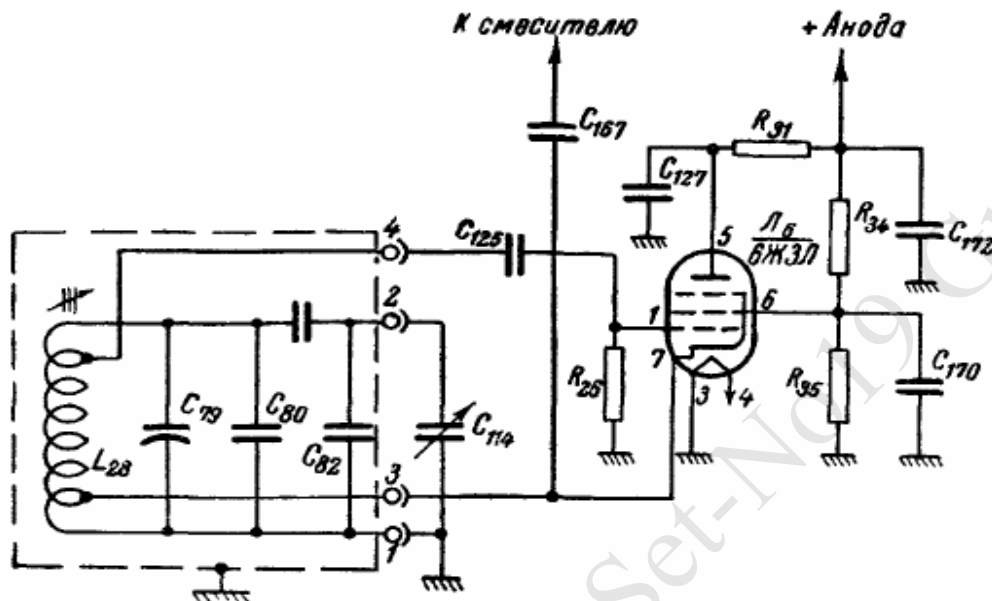
Рис. 29. Схема первого гетеродина до изменения.
