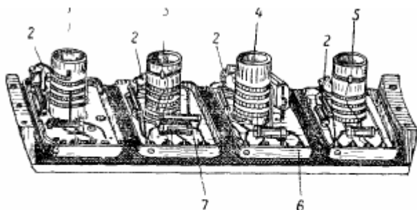
Рис. 20. Секция барабана.
