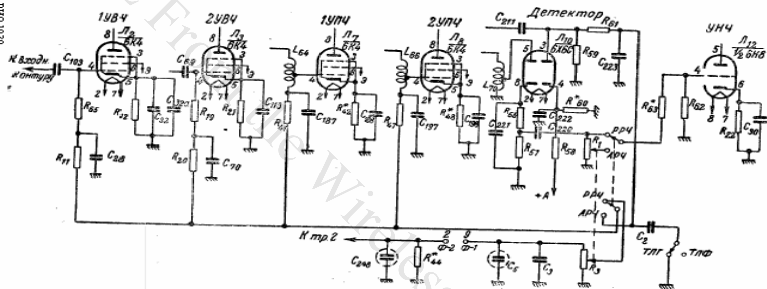
Рис. 10. Автоматическая и ручная регулировка чувствительности.
