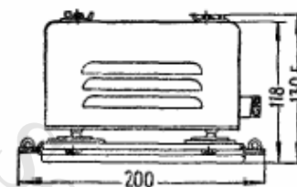
РАМА ПРИЕМНИКА
