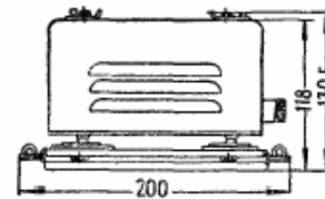
РАМА ПРИЕМНИКА
