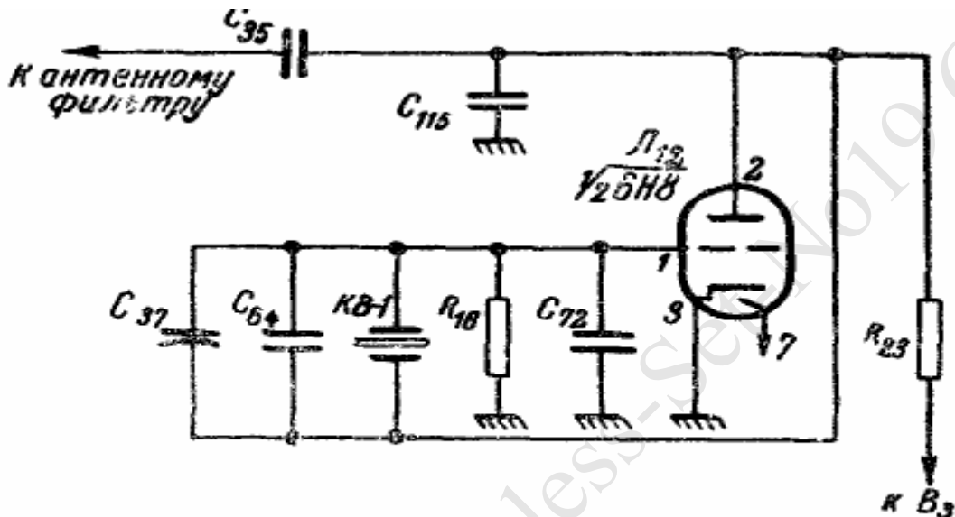
Рис. 12. Кварцевый калибратор
