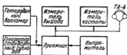
Рис. 27. Блок-схема измерения полосы пропускания приемника.
