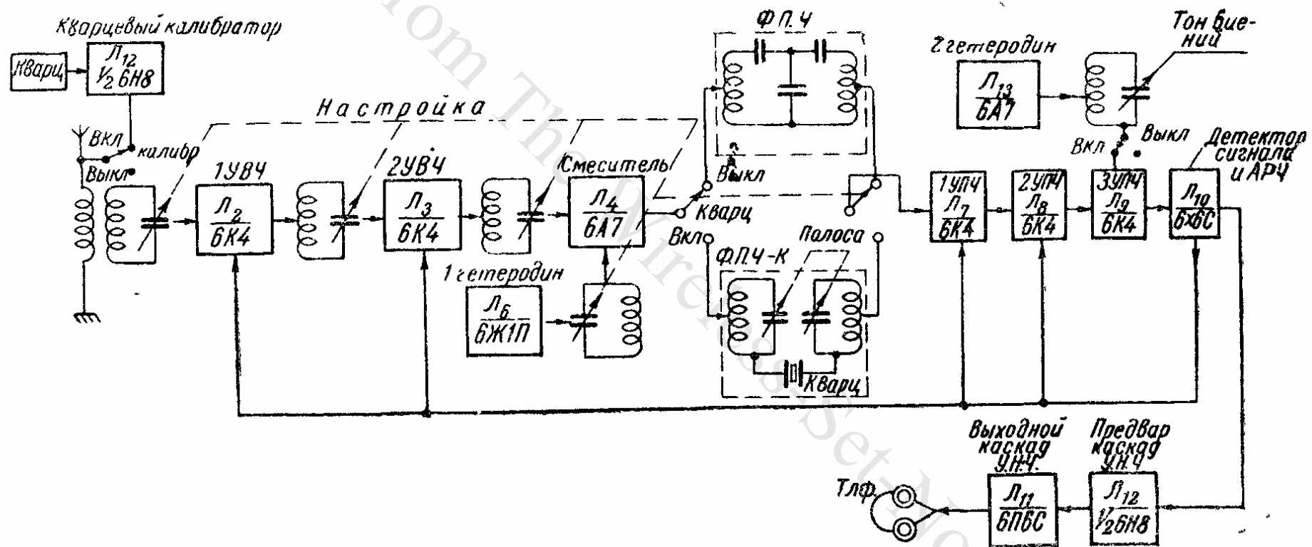
Рис. 3 Блок-схема радиоприемника.
