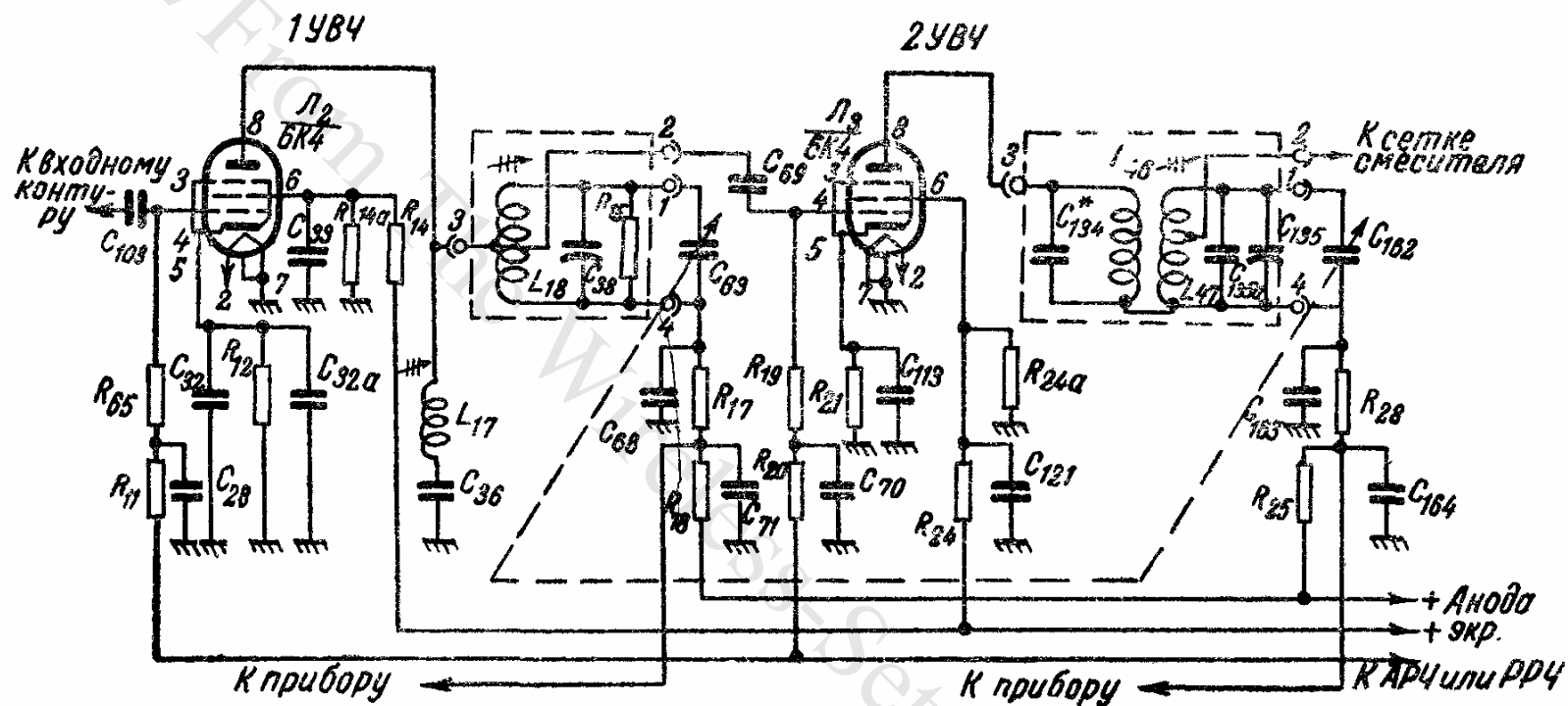
Рис 4 Усилитель высокой частоты.
