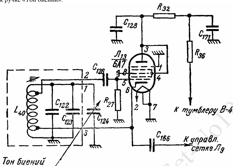
Рис. 11. Второй гетеродин
