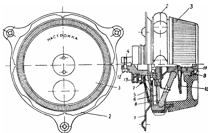
Рис. 18. Верньерный механизм
