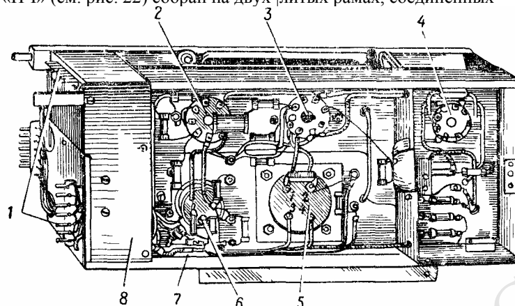
Рис. 22. Блок «НЧ»: 1—штепсельный разъем; 2—лампа L_{12} ; 3—лампа L_{11} ; 4—лампа L_{13} ; 5—выходной трансформатор; 6—кварц; 7—триммер кварцевого калибратора; 8—коробка фильтров.
