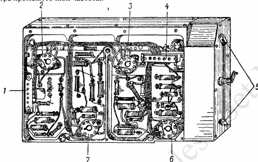
Рис. 21 Блок «ПЧ»:
