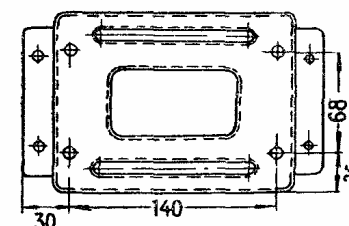
РАМА ВЫПРЯМИТЕЛЯ
