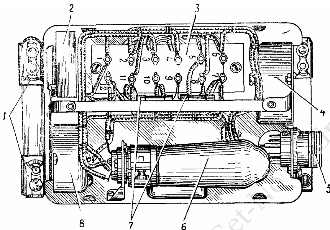
Рис 23 Блок «В»
