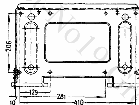
РАМА ПРИЕМНИКА
