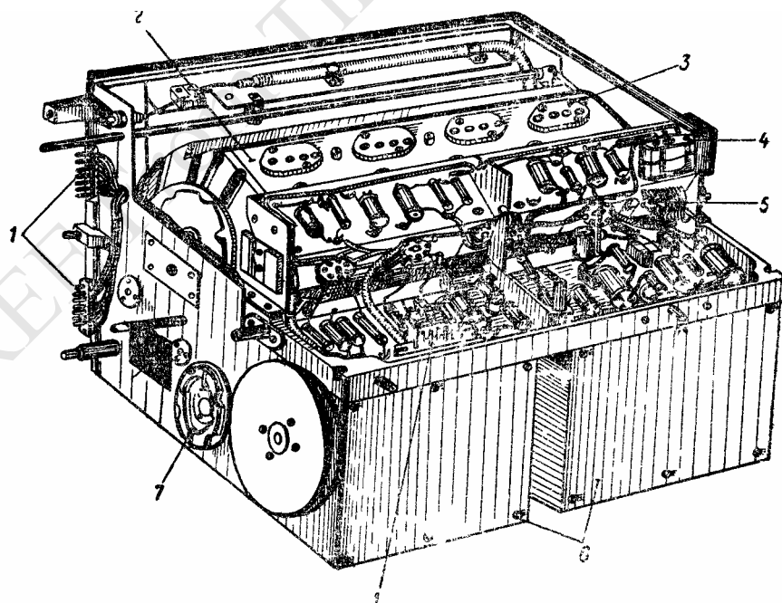
Рис. 19. Блок «ВЧ»
