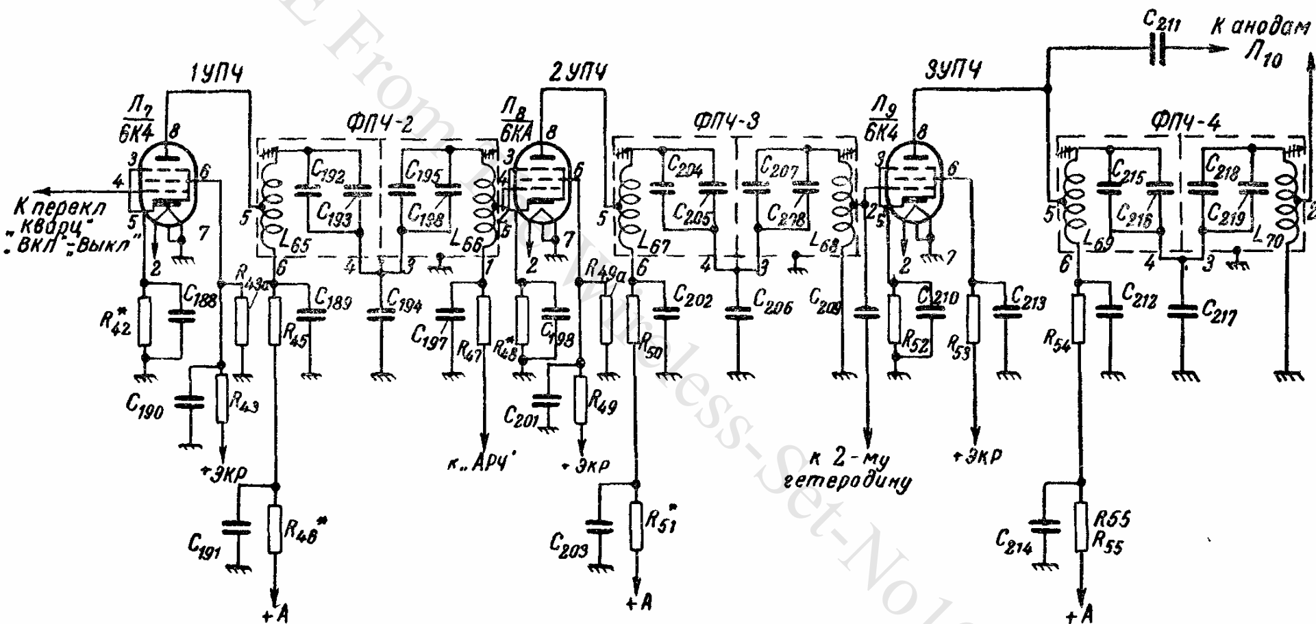
Рис. 7. Усилитель промежуточной частоты.
