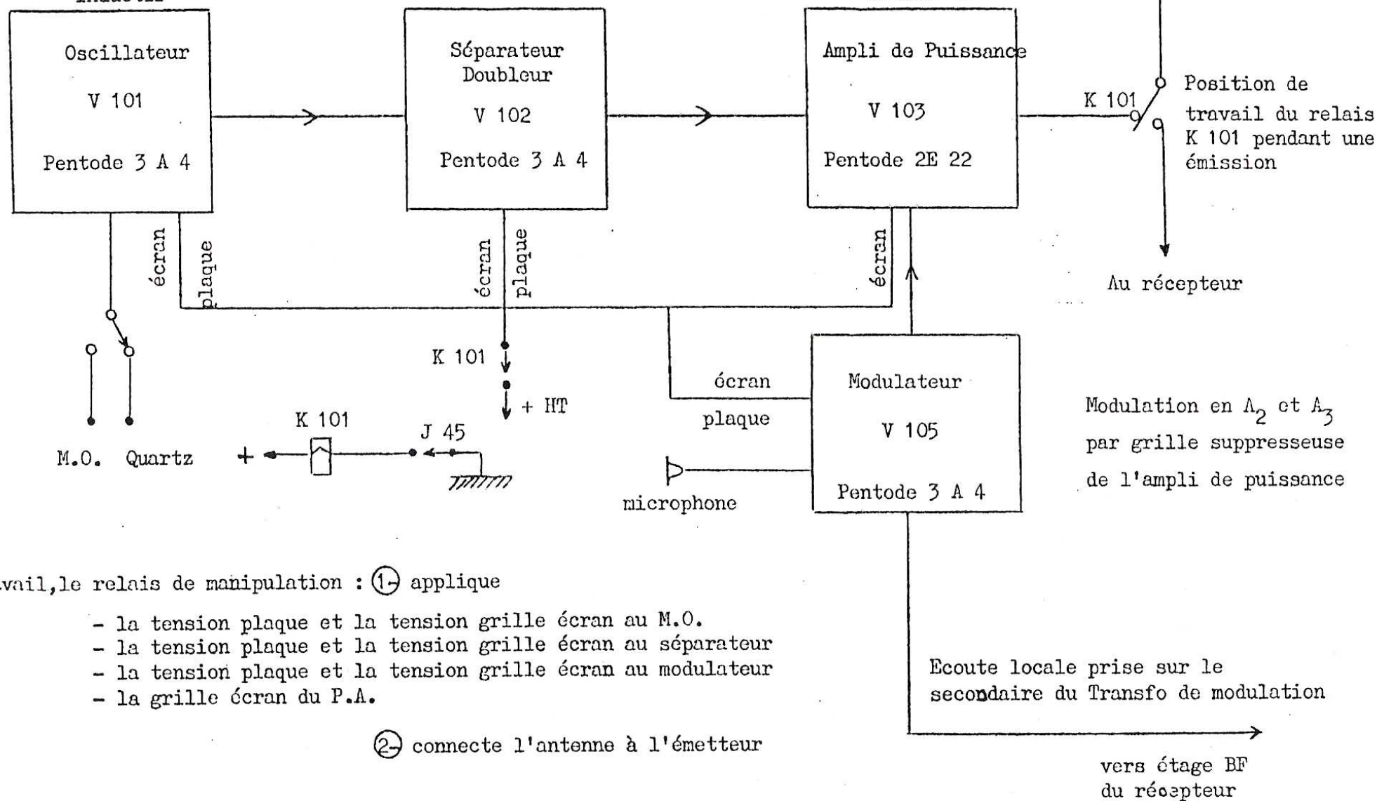
Fig. 5_Schéma simplifié de l'émetteur du RT 77/GRC.9
