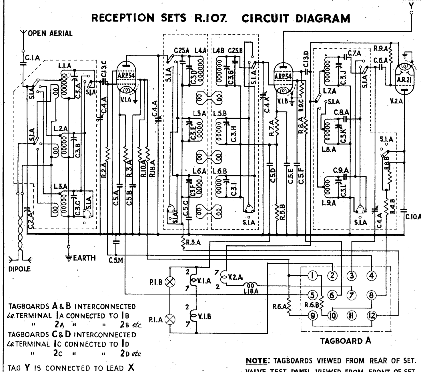
R.F. UNIT
