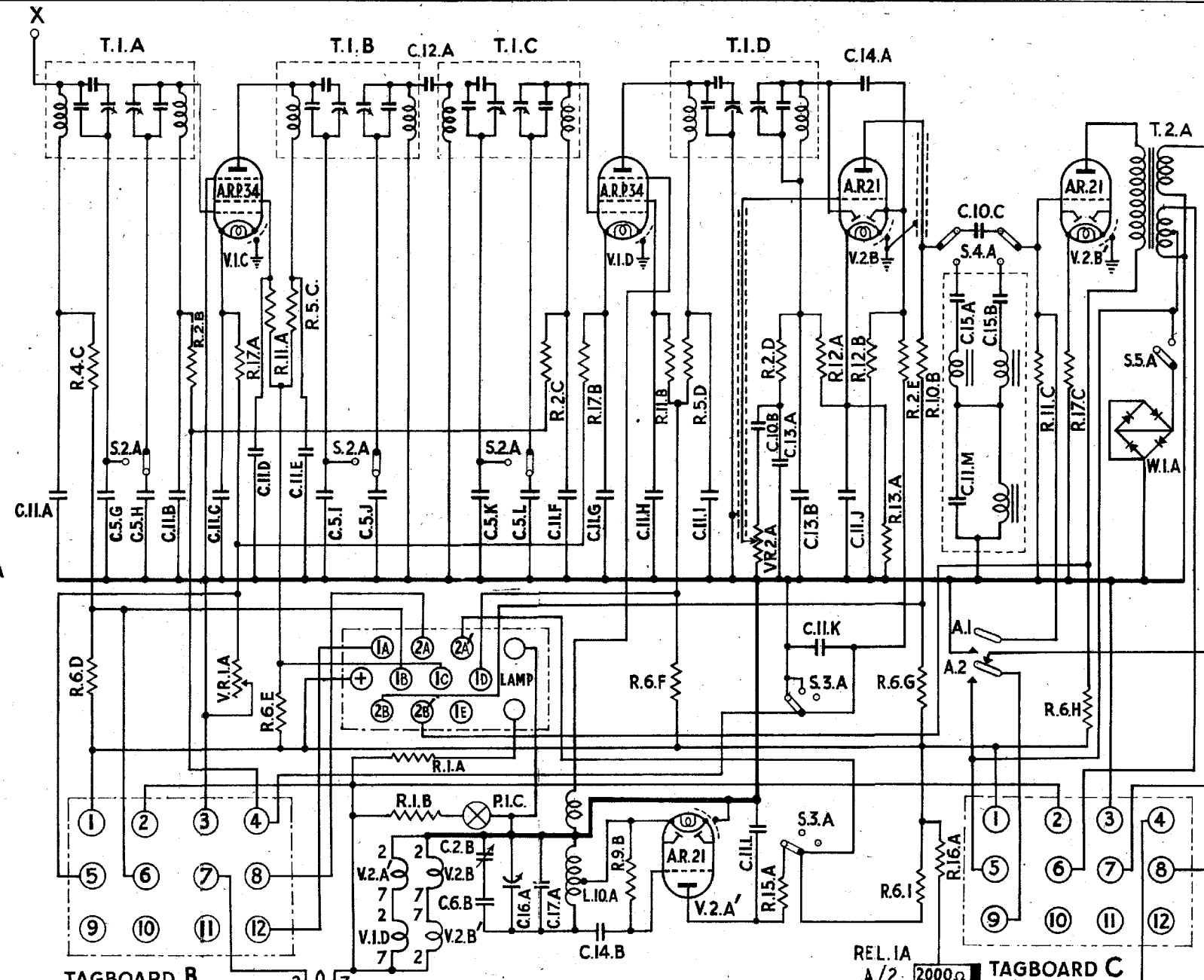
I.F./A.F. UNIT
