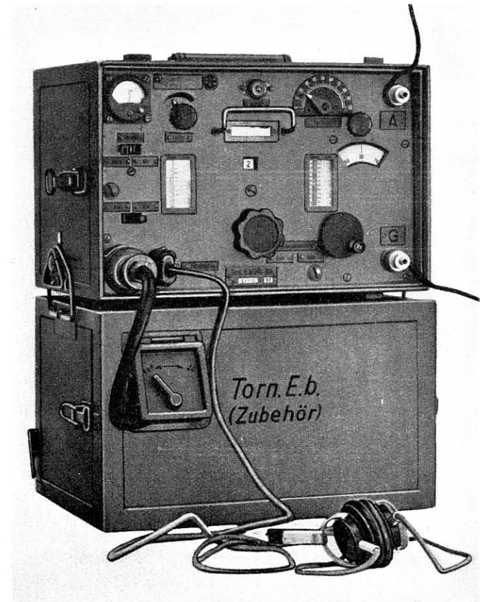
Törnister-Empfänger b (betriebsfertig)
