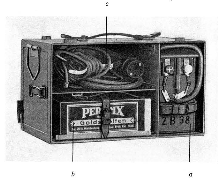
Zubehör: Halbtornister (offen)
