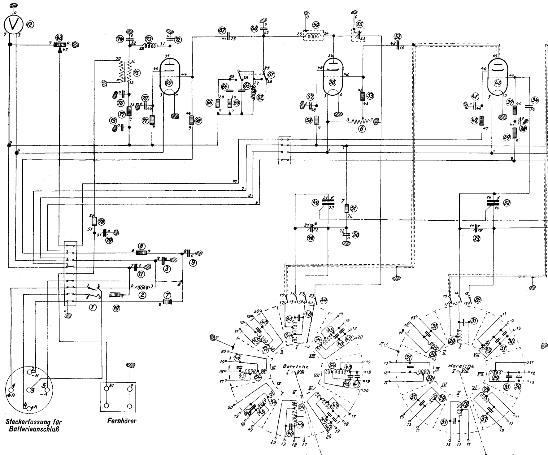
Spulentrommel für Audionstufe
