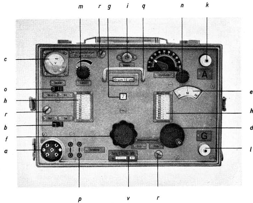
Empfänger: Halbtornister (offen)
