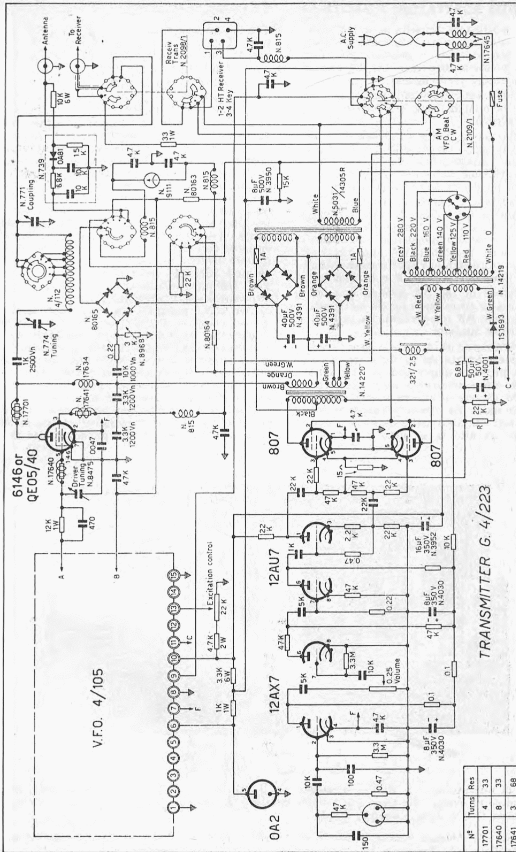
Fig. 2 - Schema elettrico del G 4/223. Lo schema particolareggiato del VFO N. 4/105 è a pag. 25. I collegamenti A e B fanno capo al commutatore di del VFO com'è indicato negli schemi a pag. 30. I terminali da 1 a 15 del VFO devono essere conteggiati tenendo l'apparecchio capovolto. G 4/223 electrical diagram. The diagram of No. 4/105 VFO is on page 25. A and B connections are connected to output selector switch of VFO, as indicated on the diagrams on page 30. VFO terminals from 1 to 15 must be counted with upset set.
