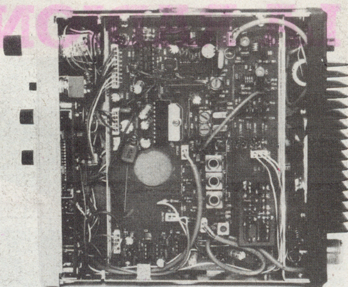
Vue du circuit imprimé supérieur.
