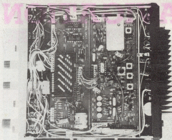
Vue du circuit imprimé inférieur : micro-processeur vers l'avant, PLL vers l'arrière.
