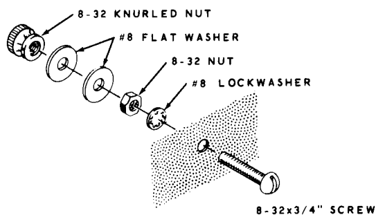
Detail 8-1E
