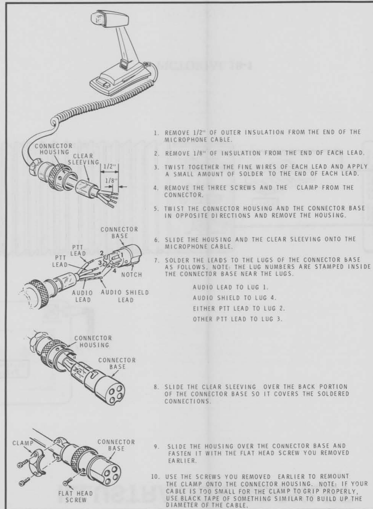
Detail 18-1C
