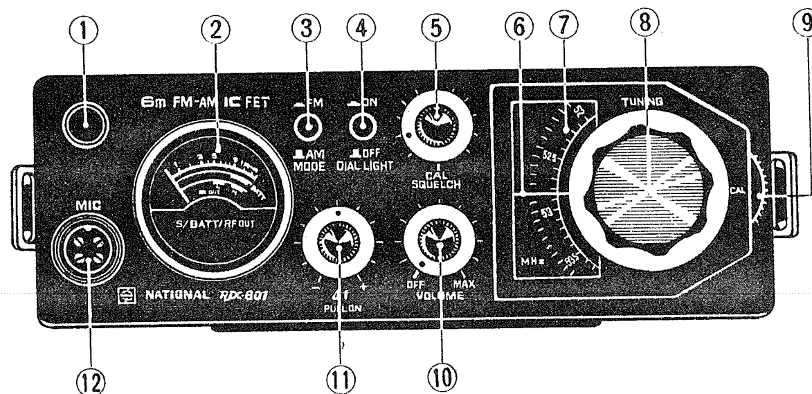
(上 面)
