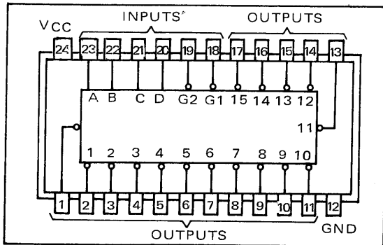
SN74159
