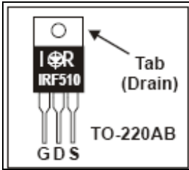
Identificación de patillas del IRF510
