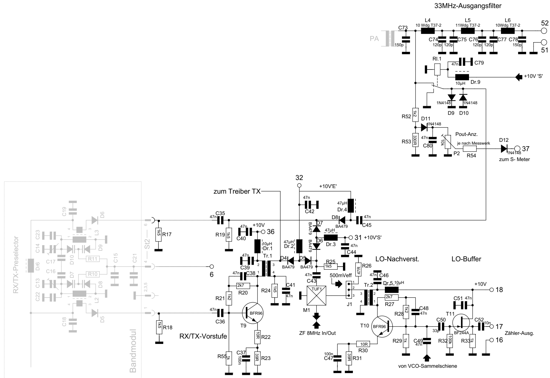
Gruppe 9 RX/TX Vorstufen, Mischer, Zählerausgang, Tiefpass
