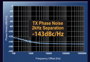
送信フェーズノイズ (14MHz帯、TX 100W、Mode: CW)
