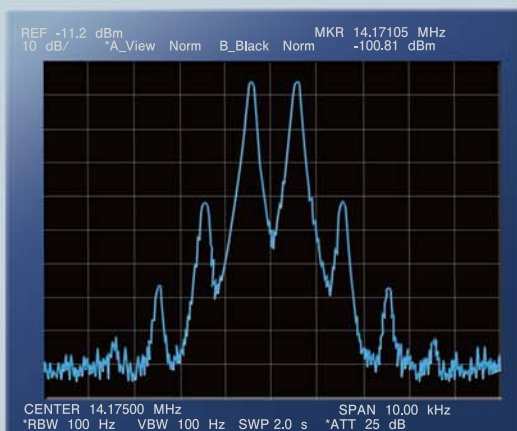
Class-A
